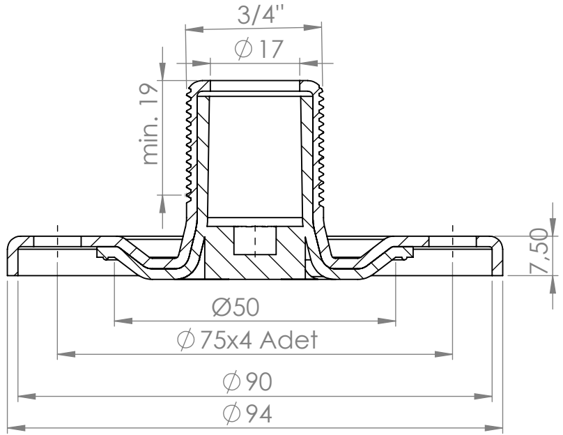
KESİT A-A ÖLÇEK 1:1
